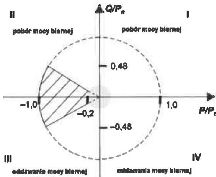
Rys.2. Zdolnořć do generacji mocy biernej w obciŹżeniowym układzie odniesienia
