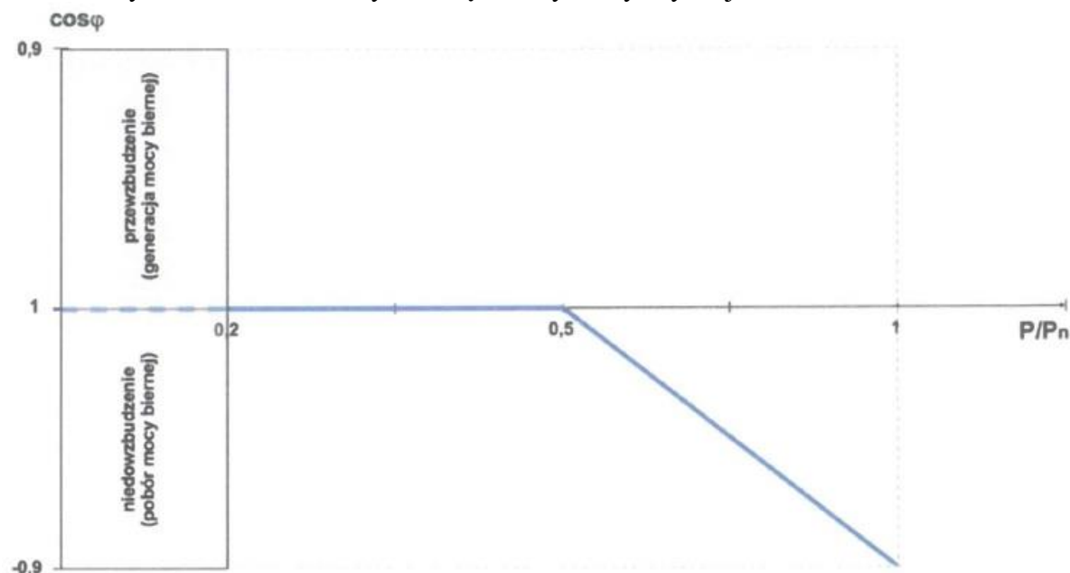
Rys.5. Charakterystyka sterowania wsp łczynnikiem mocy \cos \varphi w funkcji generowanej mocy czynnej wymagana przez OSDn.
