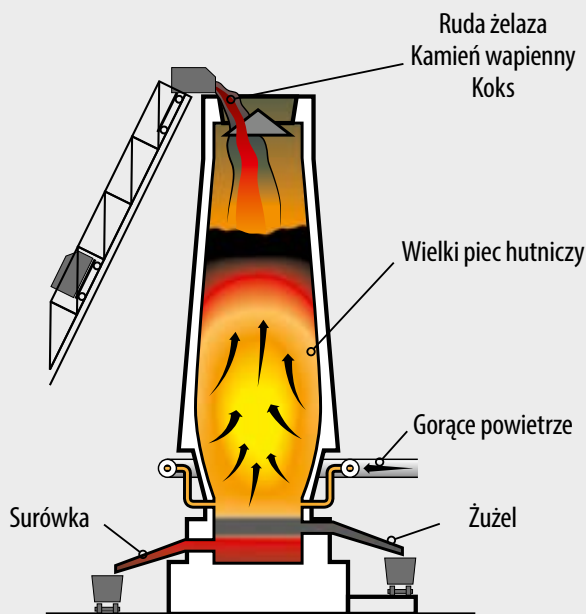
Rys. 1. Schemat wytwarzania płynnego żużla wielkopiecowego podczas wytopienia surowki w wielkim piecu hutniczym
