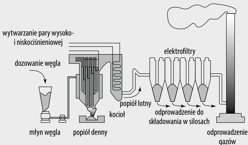
Rys. 3. Schemat otrzymywania popiołów lotnych
